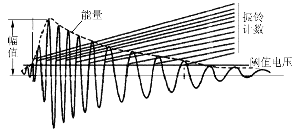
图 6 声发射信号简化波形参数定义
