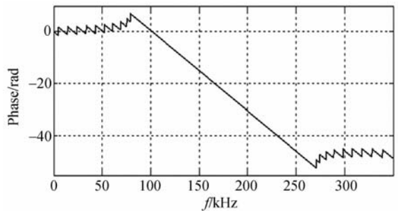
图 4 有限冲激响应滤波器相位-频率图
