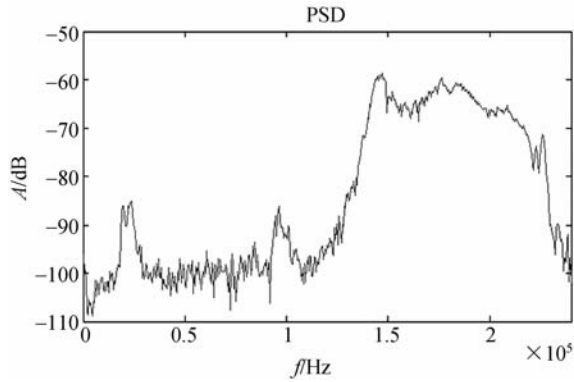
图 5 滤波后的金属裂纹声发射信号幅值-频率图
