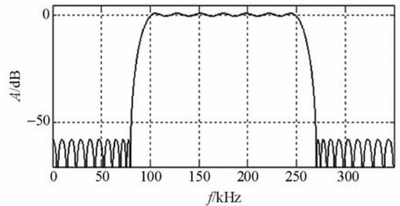
图 3 有限冲激响应滤波器幅值-频率图
