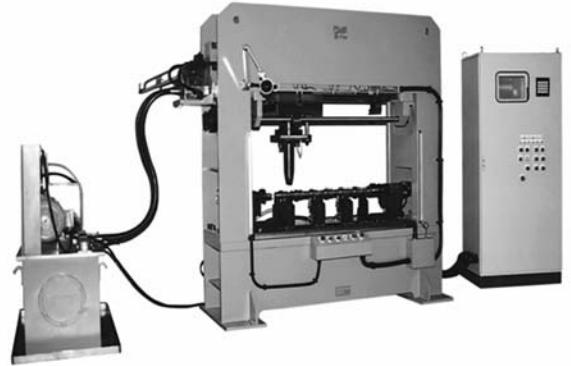
图 8 配合试验的校直机
