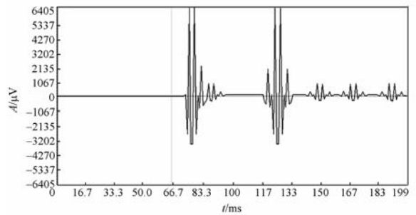
图1 金属裂纹声发射信号时域图
