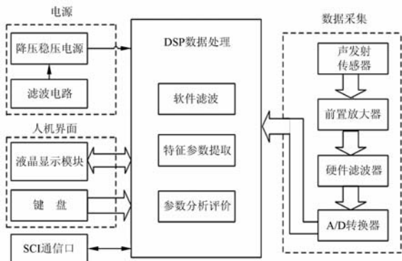
图 2 AE 实时监测系统结构框图
